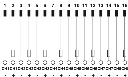
Схема подключения FLKM 16/AO/SI/DV
