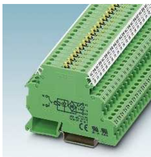
Релейные клеммные модули с выключателями
