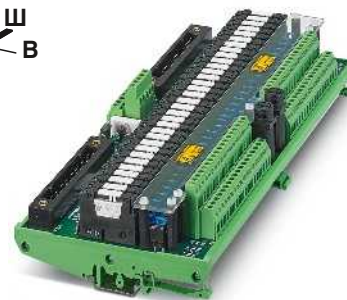
Релейный модуль вывода 230 В перем. тона
