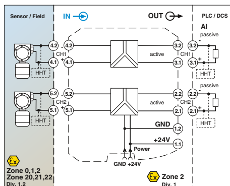
2-канальный разделительный усилитель с развязкой цепи питания
