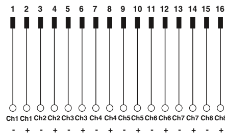
Схема подключения FLKM 16/DV
