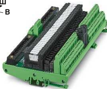
Релейный модуль вывода 24 В пост. тона
