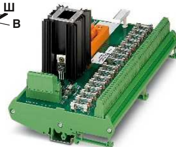
Пассивный интерфейсный модуль
