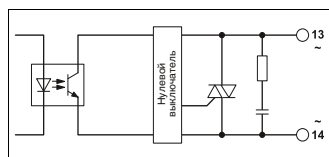
Рис. 5: Принципиальная схема, выход перемен. тока
