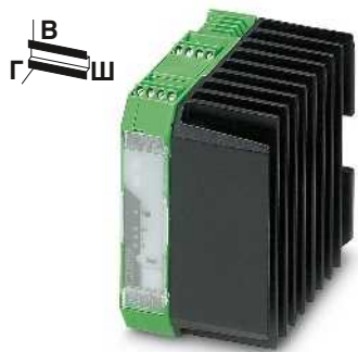
для реверсирования 3-фазных двигателей переменного тока до 575 В перем. тока/3 x 9 A
