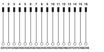
Схема подключения FLKM 16/AI/DV
