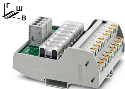
с зажимом push-in, 2 потенциала и восемь предохранителей 6,3 А
