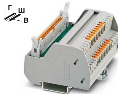
Соединительный модуль VARIOFACE для 16 каналов с зажимами Push-in
