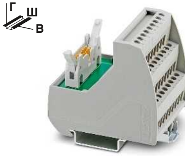
Модули инициатора с винтовыми зажимами
