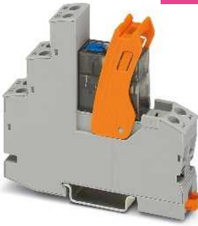
Релейный модуль с 2 переключающими контактами с винтовым зажимом и ручным управлением
